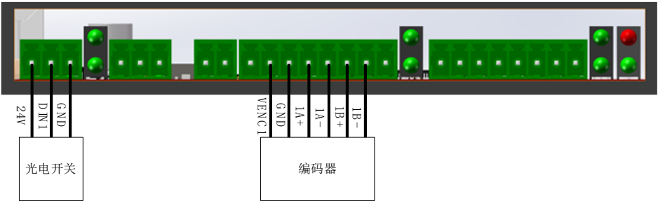
图 5 接线示例
